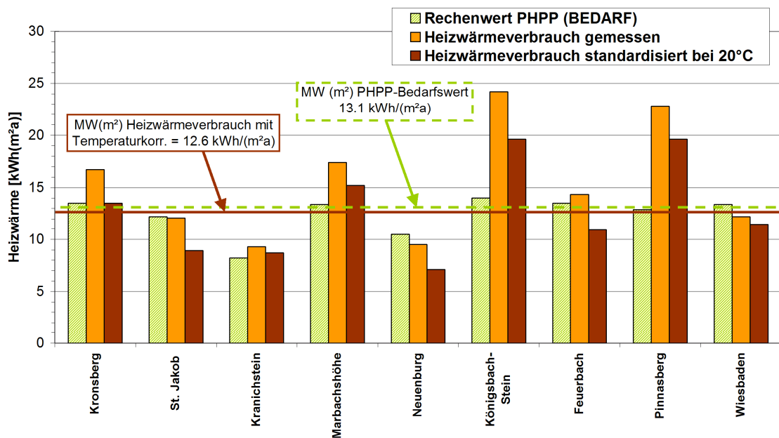
Abbildung 7: Gemessener Heizwärmeverbrauch im Vergleich mit dem Projektierungswert von Reihen-, Doppel- und Mehrfamilienhäusern im Passivhaus Standard. Der PHPP Rechenwert ist für 20°C Raumtemperatur berechnet worden (aus [Peper 2008])
